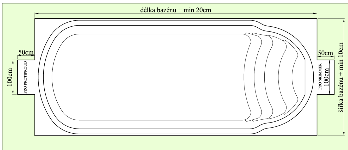
půdorys výkopu
