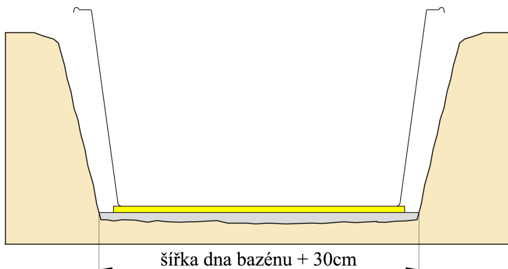
příčný řez výkopem - šířka betonové desky dle typu bazénu
