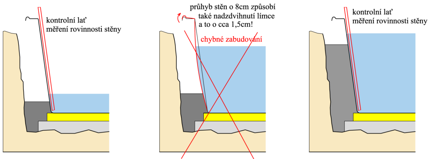
kontrola rovinnosti stěn ve svislém směru
